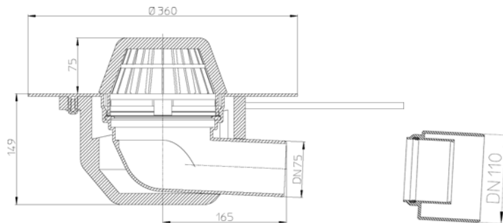
Рис. 1. Кровельная воронка HL64.1P.
