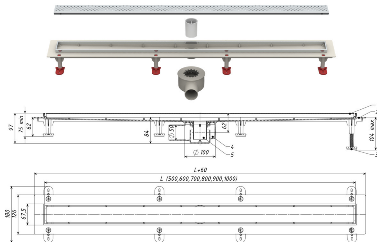
Рис. 1 – Габаритные размеры
